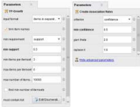
Figura 2. Configuración de los parámetros de entrada para el algoritmo FP-Growth . Finalmente, se obtuvieron reglas de asociación en formato tabular, gráfico y en descripción lógica, como se muestra a continuación, comenzando por la Figura 3.
