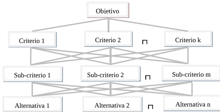
Figura 1. Esquema en forma de árbol sobre los elementos necesarios para aplicar la técnica AHP .
