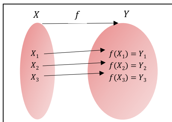
Ilustración 147: Función biyectiva
