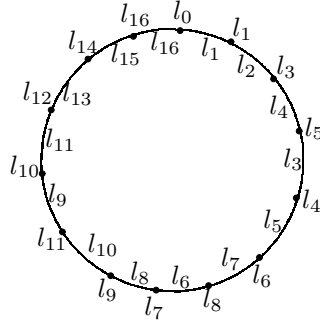
Fig.3.3 C_{14}
