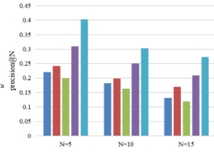
(b)precision@N
