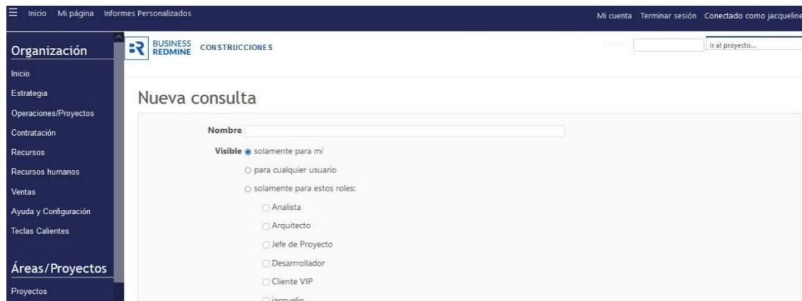
Figura 56. Nueva consulta
