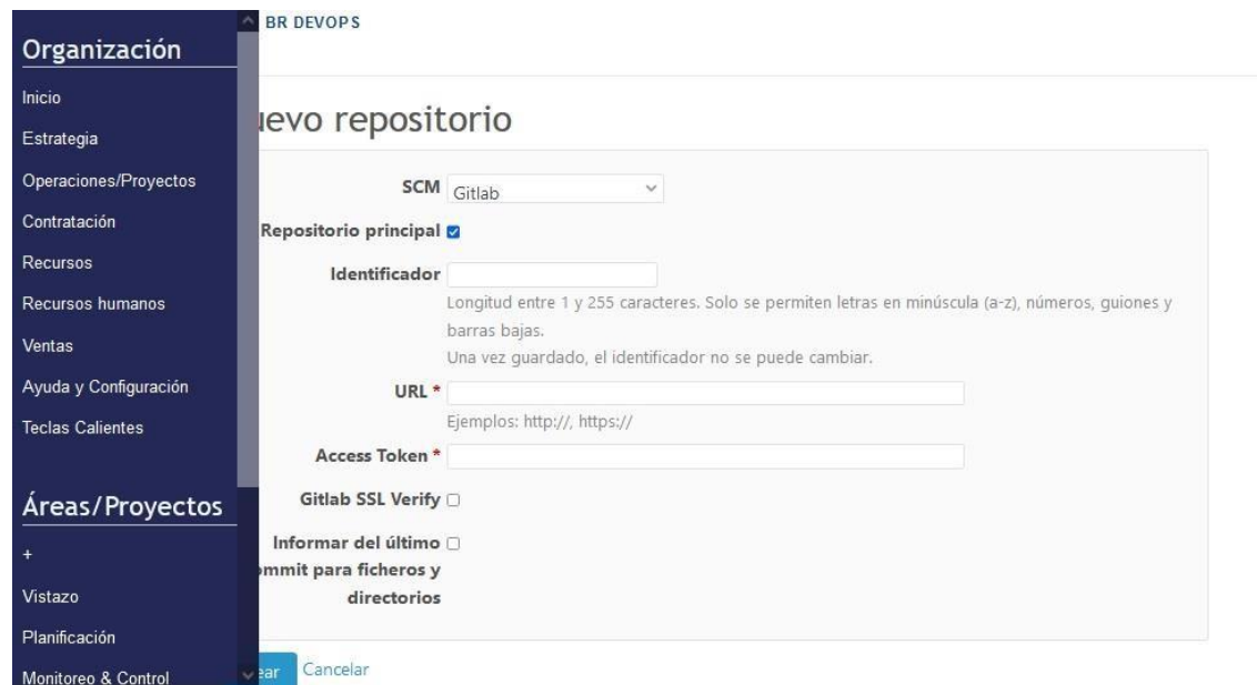
Figura 290. Nuevos repositorios.
