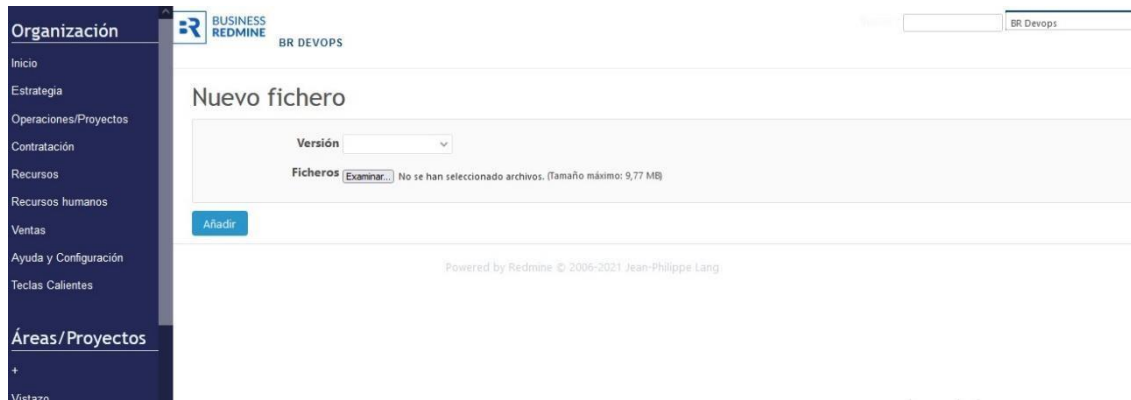
Figura 86. Nuevo fichero
